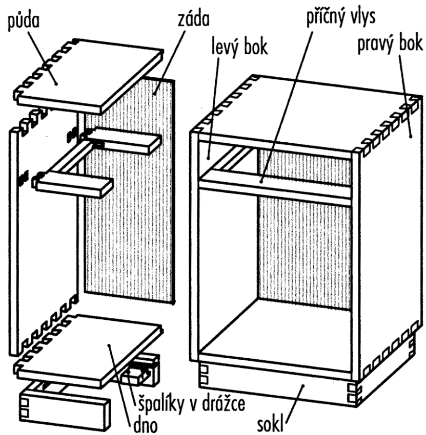
Jednoduchý korpus dosková konstrukcia (přírodní dřevo)
