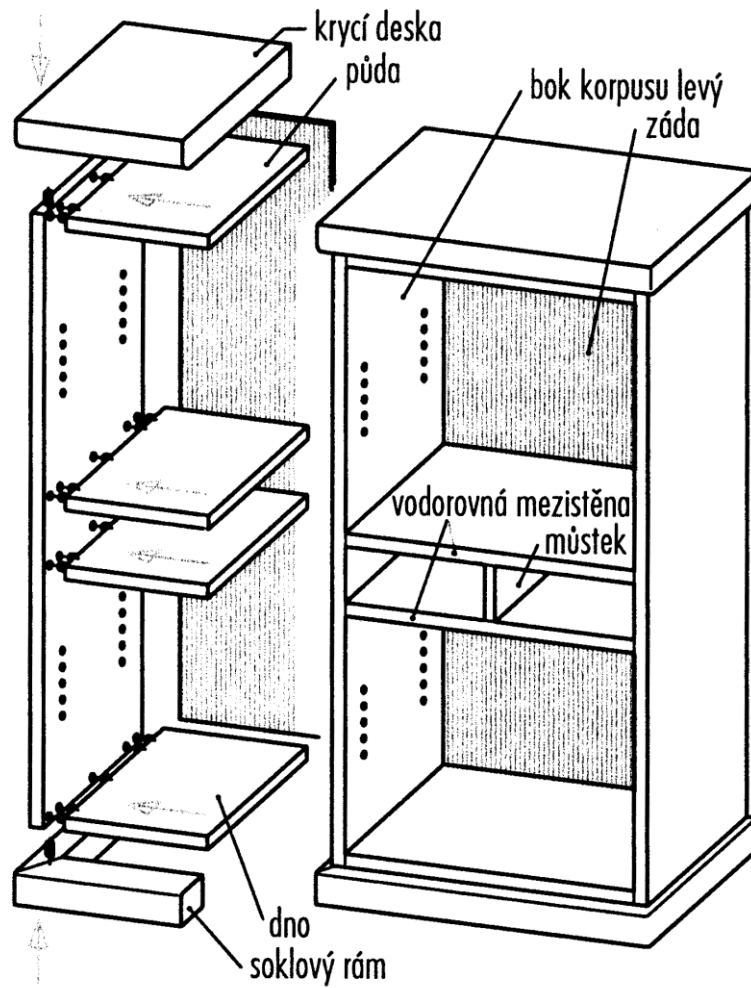
Korpus s vrchnou krycí doskou
