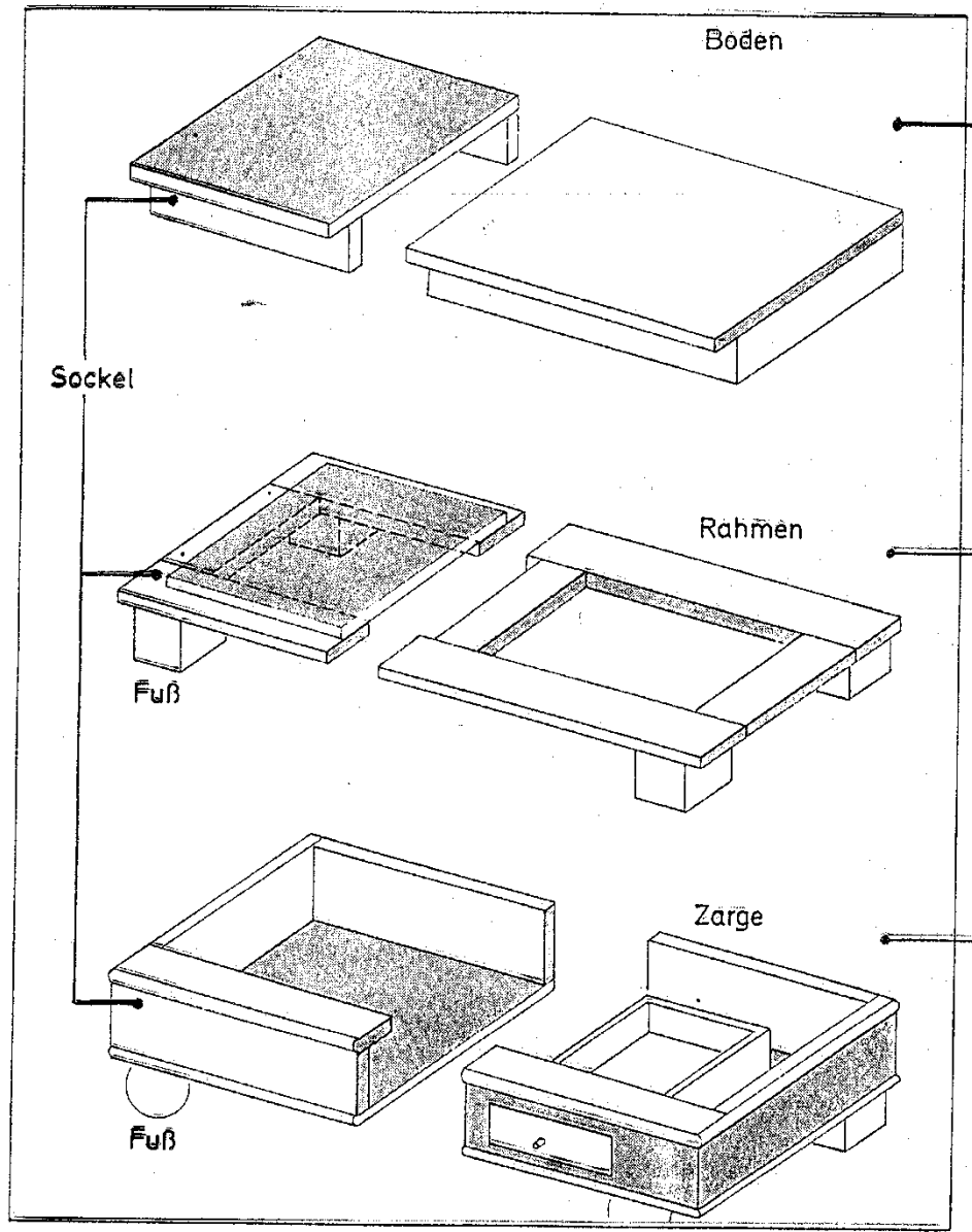
Korpus s (funkčným) soklom a vencom (historické konštrukcie)
