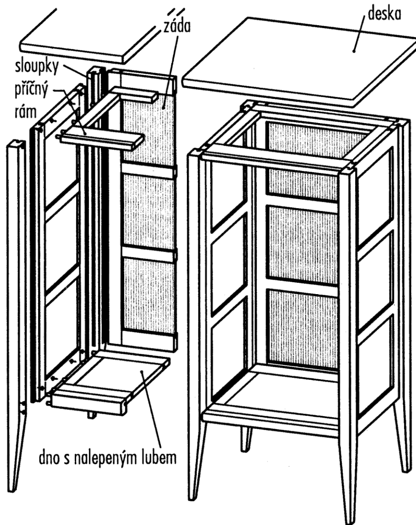
Stípková konštrukcia – stípičky a výplne
